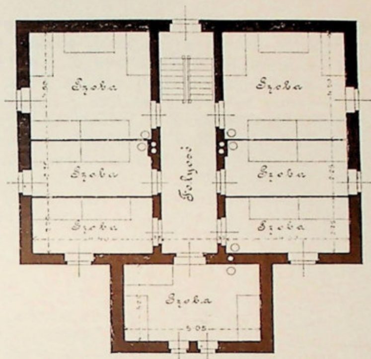
Az új Bárá Eötvös Loránd-menedékház emeleti alaprajza.
