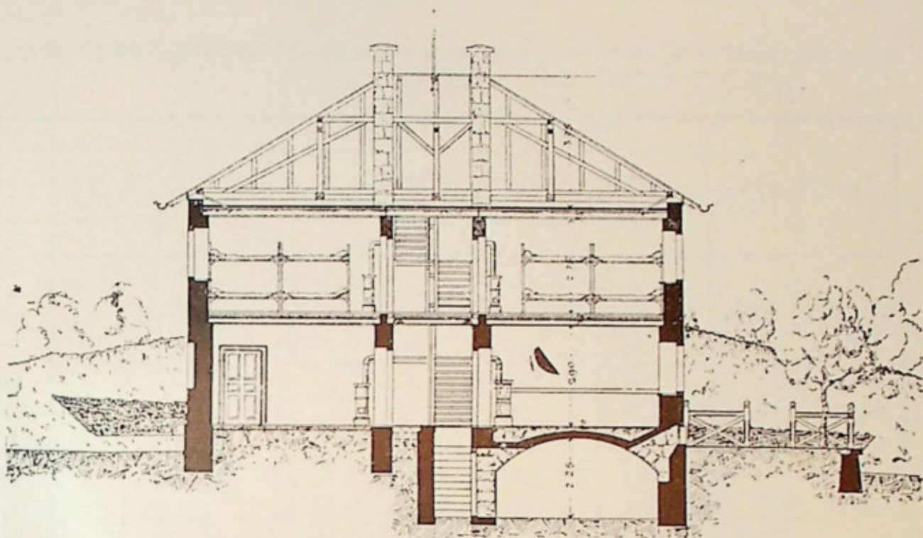
Az új Bárá Eötvös Loránd-menedékház keresztmetszete.
