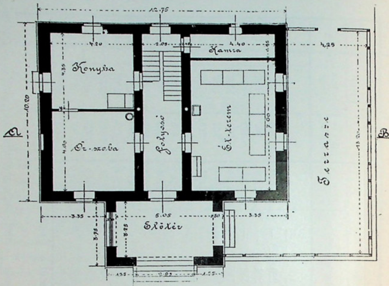
Az új Báró Eötvös Lóránd-menedékház földszinti alaprajza.
