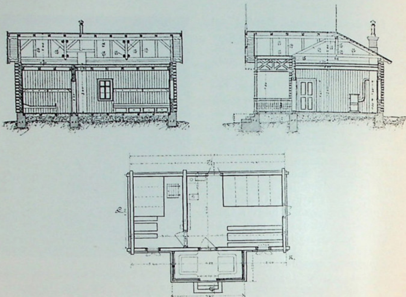
A dobogókői régi Báró Eötvös Loránd-menedékház alaprajza és keresztmetszetei.
