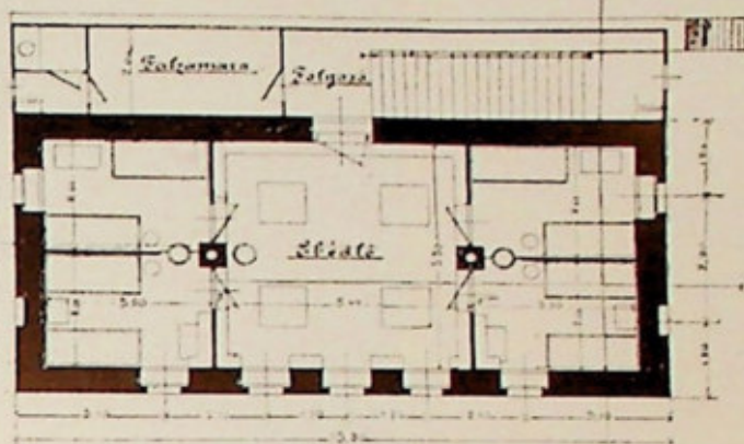
A Térvényház emeleti alaprajza.
